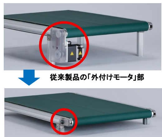
モータをコンベヤ内部に格納する新設計
